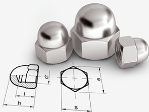
مهره سرپشته Hexagon Domed Cap Nuts DIN 1587
